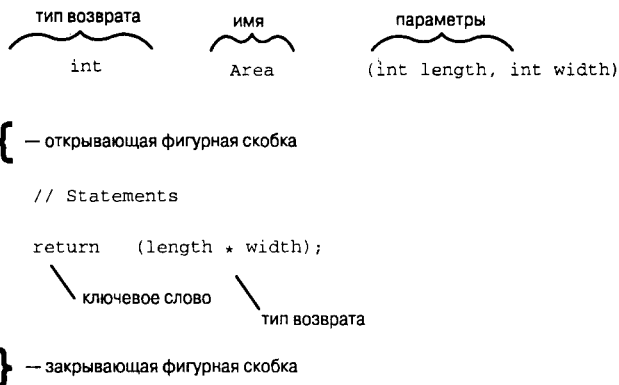
Рис. 5.3. Заголовок и тело функции
