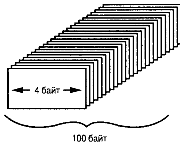
Рис. 12.1. Объявление массива
