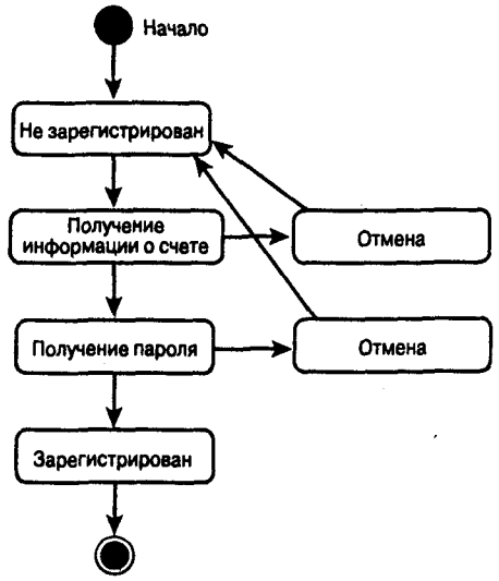
Рис. 18.24. Отмена регистрации
