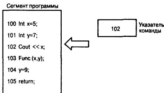
Рис. 5.6. Указатель команды
