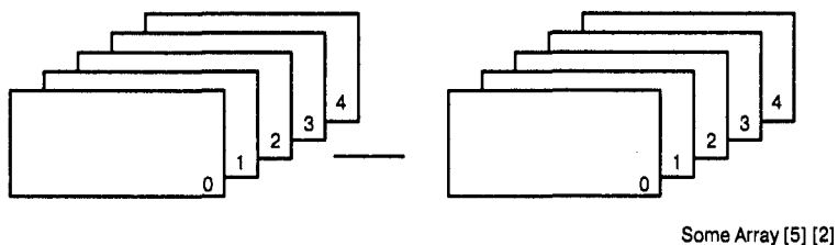
Рис. 12.4. Массив 5×2
