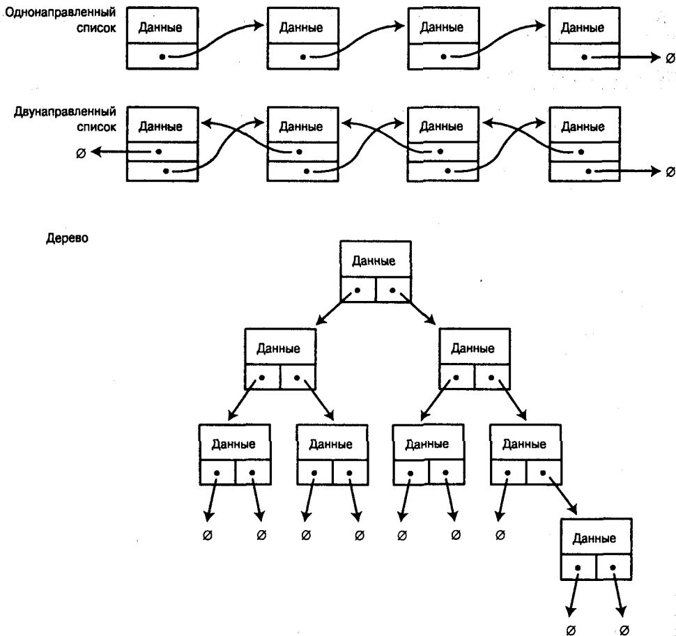
Рис. 12.5. Связанные списки
